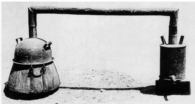
Նկար 23գ. Օղի թորելու սարք (1967 թ.), Էջմիածին (ՀՀ ԳԱԱ հնագիտության և ազգագրության ինստիտուտի ազգագրության բաժնի արխիվ)
