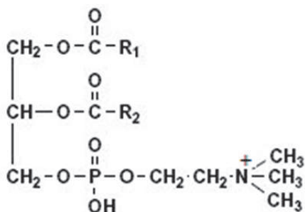
ֆոսֆատիդիլսոլին
