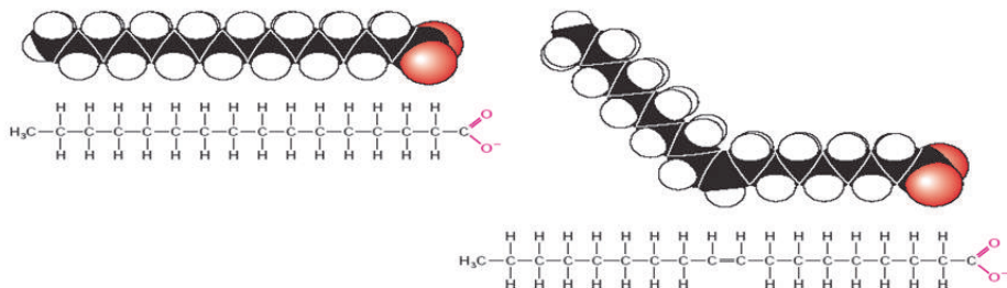
հազեցած պալմիտինաթթու
