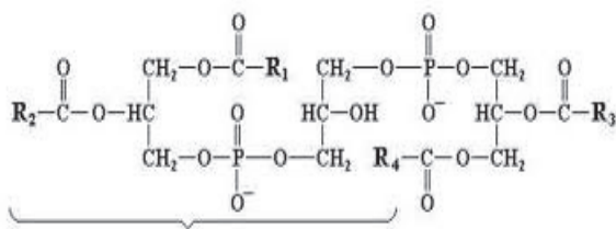
ֆոսֆատիդիլգլիցերոլ
