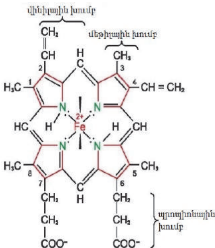
հեմոգլոբին
