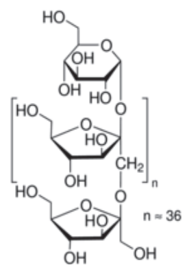
Ինուլին
