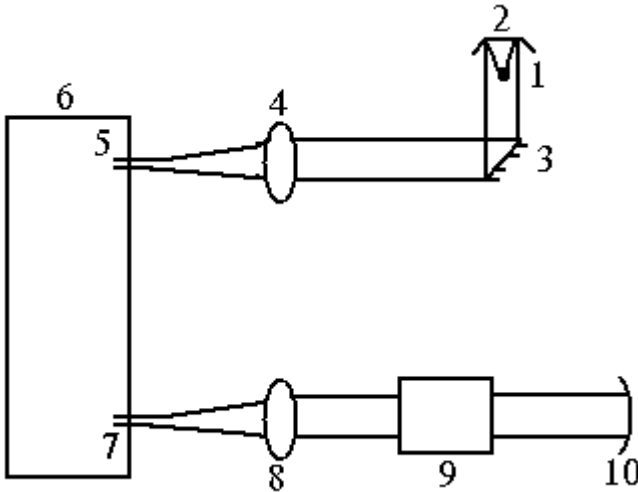
Նկ. 1. Միաճառագայթ սպեկտրաֆոտոմետրի կառուցվածքային գծապատկերը:
