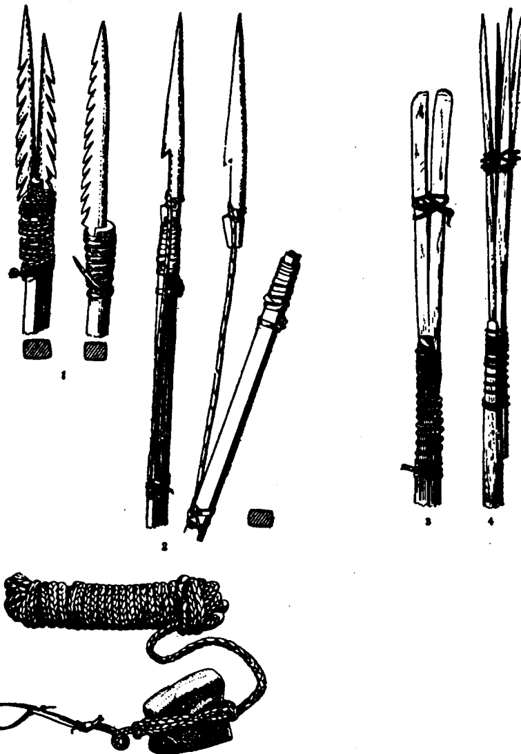
Հրոերկրիցիների գործիքներ. 1 - նիզակներ, 2 - տեգեր, 3 - կակղամորթների որսի գործիք, 4 - ծովախեցգետինների որսի գործիք, 5 - «կարթ»
